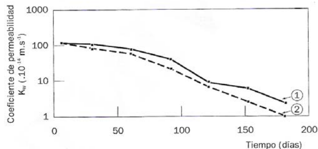
Figure 1C.2. - Evolución del coeficiente de permeabilidad al agua de un hormigón proyectado de cemento natural PROMPT con el envejecimiento.
